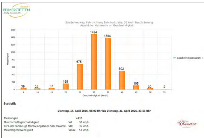
Auswertung Heuweg (Fahrtrichtung Bahnhofstraße) 14.04. - 21.04.2026
